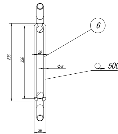
PRZEKRÓJ Y-Y SKALA 1 : 7
